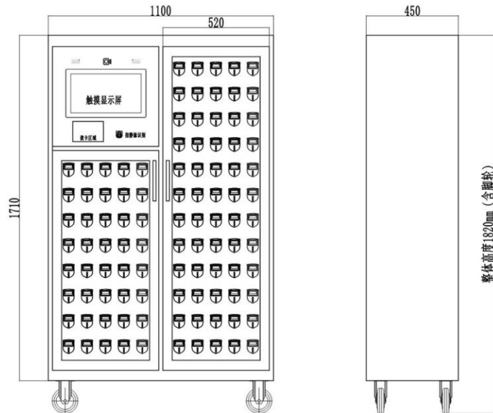
(产品尺寸图)
